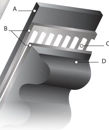
A : Protección de alta resistencia B : Mezcla de unión específica de EPDM C : Cable de alta resistencia, poco estiramiento (poliéster reforzado endurecido) D : Mezcla de EPDM reforzada con fibras orientadas
